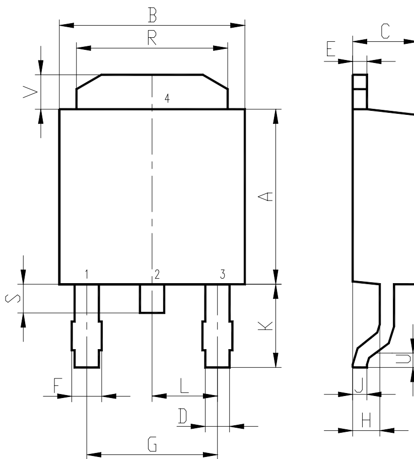
КТ-89 (DPAK)
