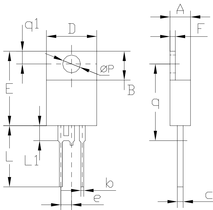
КТ-28-1 (ТО-220АС)
